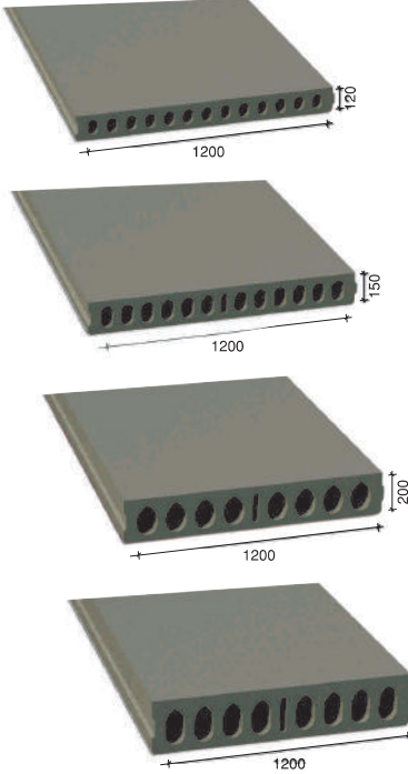
örnek kesit tipleri ve boyutlar
