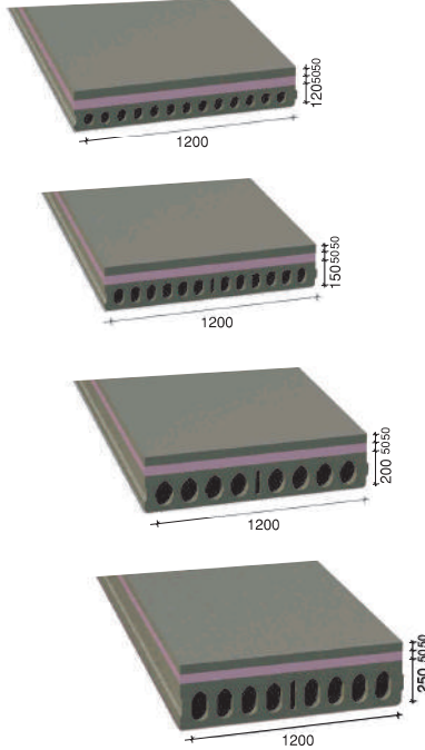
ısı yalıtımlı kesit tipleri
